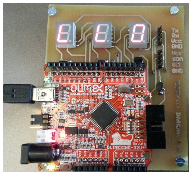
FIGURE 4 – Affichage d'un message défilant sur les afficheurs 7-segments. À gauche les lettres HEL, à droite LLO.
