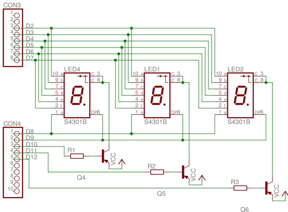
FIGURE 2 – Schéma de principe de la carte 7-segments.
