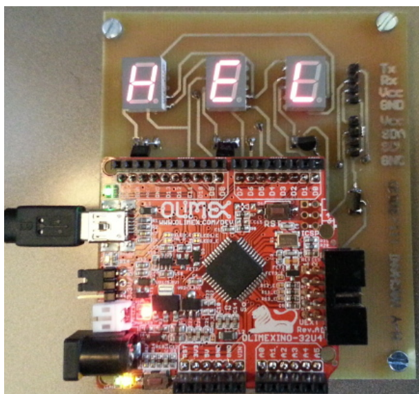
FIGURE 4 – Affichage d'un message défilant sur les afficheurs 7-segments. À gauche les lettres HEL, à droite LLO.
