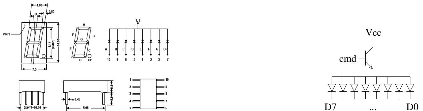
FIGURE 1 – Gauche : extrait de la datasheet d'un afficheur 7-segments, repris de http://datasheet.sparkgo.com.br/LD3361BS.p . Droite : câblage interne à l'afficheur 7-segments.
