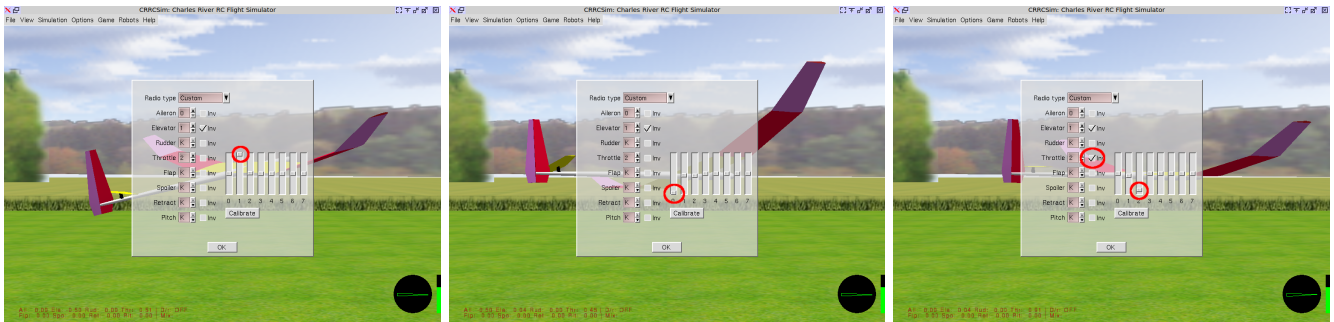
FIGURE 7 – Test des diverses commandes de l’avions par le menu Options → Controls → Configure : de gauche à droite, le lacet (canal 1), le tangage (canal 2) et la puissance moteur (canal 3) après avoir inversé cette commande pour tenir compte du câblage de l’alimentation et masse aux bornes de ce potentiomètre.
