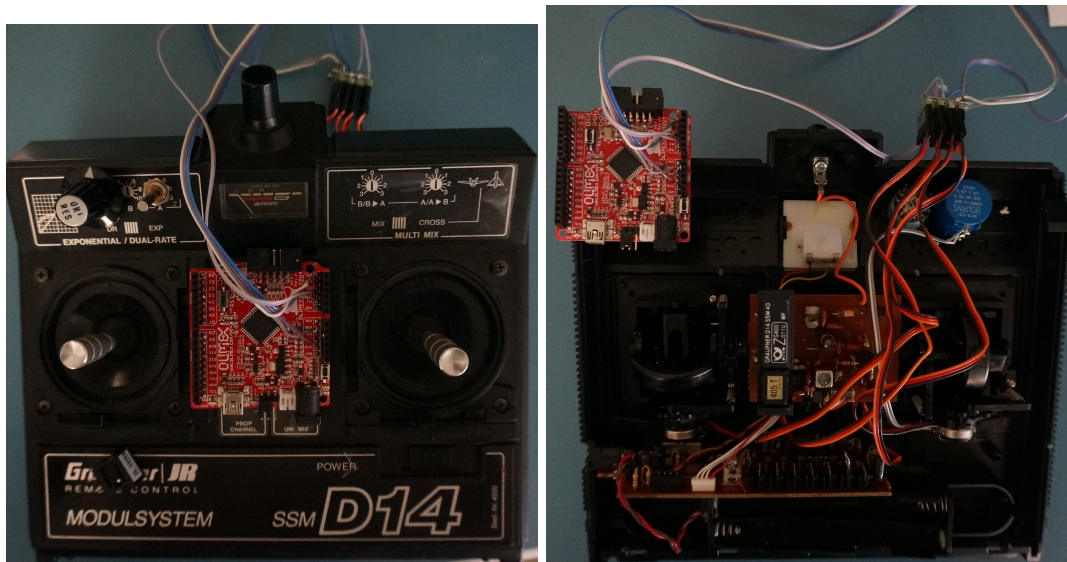
FIGURE 4 – Connexion du microcontrôleur à la radiocommande : l'électronique interne est déconnectée, seuls les potentiomètres sont connectés aux extrémités à la masse et tension d'alimentation, et le point milieu sur chaque entrée de convertisseur analogique-numérique. Aucun dommage irréversible à la radiocommande n'est nécessairement nous n'avons fait que déconnecter les nappes venant des manettes pour les connecter au microcontrôleur.
