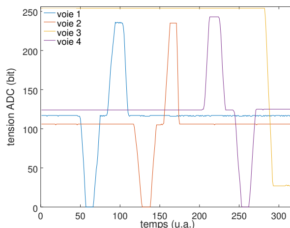
Figure 5: Conversion des valeurs brutes au format FMSPIC : les données sont cette fois codées sur 8 bits (valeurs comprises entre 0 et 255 – 254 en pratique pour ne pas confondre avec l'octet de synchronisation de trame) et exploitent toute la gamme de mesure.
