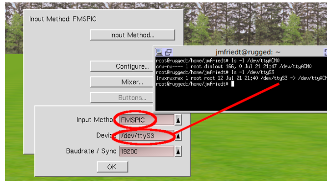
FIGURE 6 – Lien symbolique entre l’interface émulant le port de communication asynchrone sur USB /dev/ttyACM0 avec une des ports série prévus dans CRRCSim, ici arbitrairement /dev/ttyS3 .
