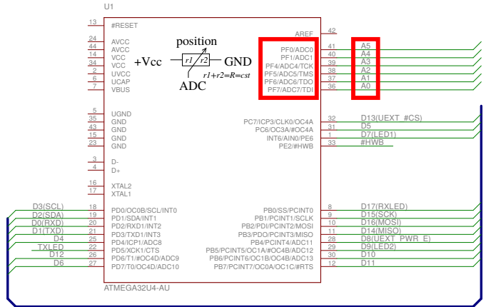
Figure 2: Schéma de la carte Olimexino32U4, mettant en évidence l'incohérence entre les broches du microcontrôleur et la sérigraphie du circuit imprimé. En insert dans le schéma : câblage d'un potentiomètre tel qu'utilisé pour lire la position de chaque manette. La résistance variable (point milieu) est polarisée entre la masse et la tension de référence du convertisseur analogique-numérique, ici la tension d'alimentation du microcontrôleur.
