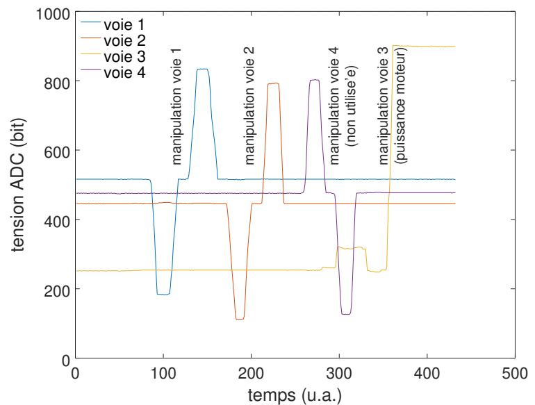
Figure 3: Tracé des mesures des diverses voies de la radiocommande, alors que chaque manette est séquentiellement manipulée entre ses valeurs extrêmes
