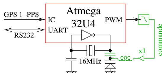
FIGURE 2: Schéma de principe, avec le 1-PPS issu du récepteur GPS qui alimente une entrée input capture (IC) connectée à un compteur ( timer ). L'écart de fréquence à la valeur nominale est corrigée en polarisant une varicap faisant office de condensateur de pieds d'un oscillateur à quartz comprenant un résonateur et la porte inverseuse se comportant comme amplificateur introduisant un déphasage de 180^\circ . Le filtre passe-bas chargé de lisser la PWM, l'amplificateur suiveur, l'inductance bloquant la fuite du signal radiofréquence et le condensateur de blocage de la commande DC vers l'amplificateur (en vert) ne seront pas explicités dans ce document qui se focalise sur les éléments numériques de l'asservissement.
