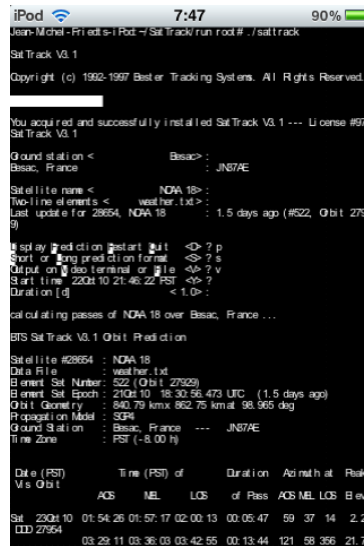
FIG. 3 – Sattrack – un logiciel de prévision de passage de satellites opensource jusqu’à sa version 3.1.6 malgré une license très restrictive – fonctionne en mode texte ( MobileTerminal ) sur iPod avec la gestion de la position du curseur au moyen des caractères de contrôle compatibles avec un terminal VT100. Cette application permet d’identifier les satellites visibles dans le ciel après le coucher du soleil, ou de prédire le prochain passage d’un satellite météorologique. Dans cet exemple, nous avons obtenu les paramètres orbitaux les plus récents sur www.celestrak.com et calculé les dates de passage du satellite en orbite basse polaire NOAA 18.
