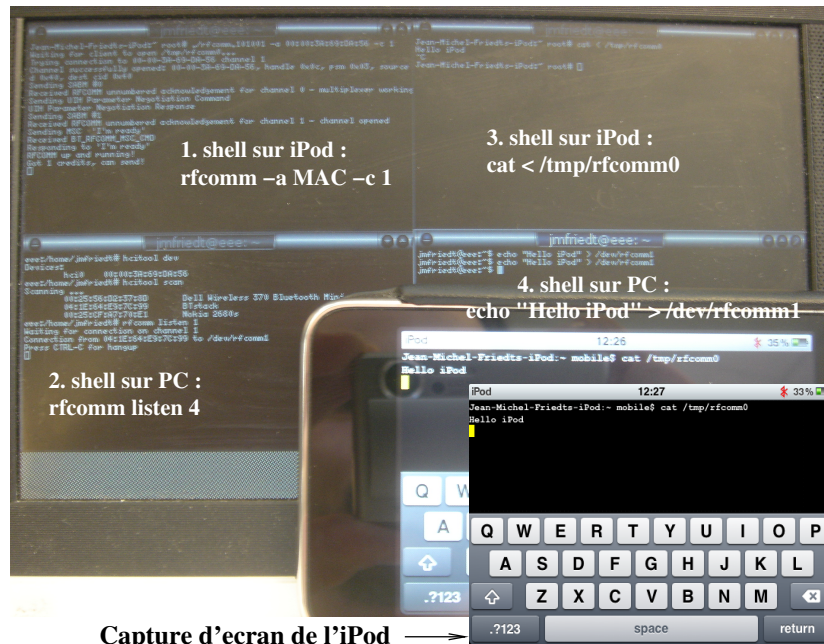
FIG. 9 – Transmission de données depuis un shell sur PC, via un convertisseur USB-Bluetooth, vers iPod, au moyen des outils rfcomm exécutés sur les deux interlocuteurs.
