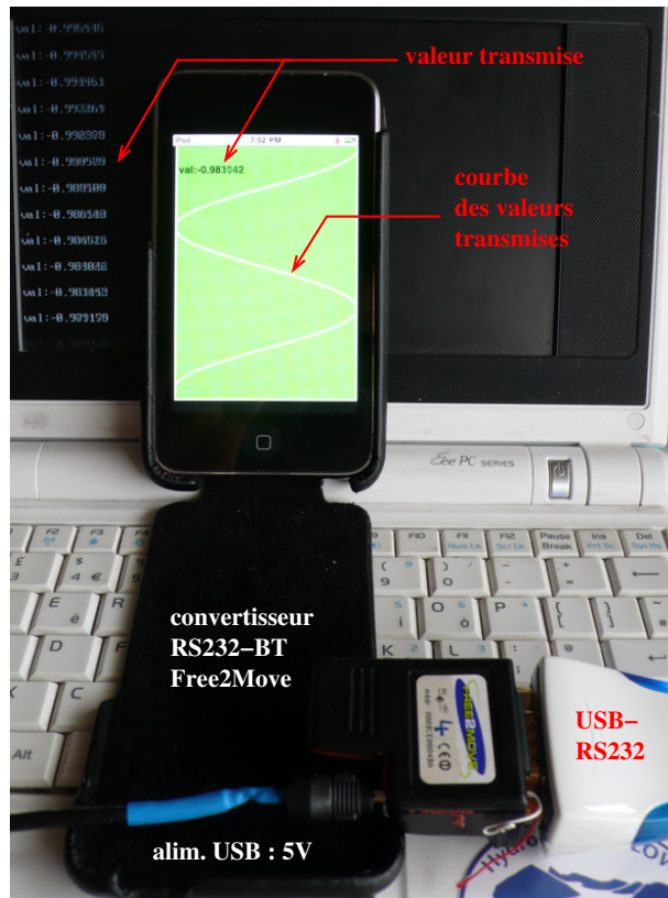
FIG. 11 – Transmission de données depuis un PC, via un convertisseur RS232-Bluetooth lui même connecté par convertisseur USB-RS232, pour affichage sur iPod. Cette application est représentative d'une application dans laquelle les données sont acquises par un microcontrôleur et transmises par liaison Bluetooth grâce au convertisseur Free2Move, les données étant émises selon un format val : valeur au travers du port série.
