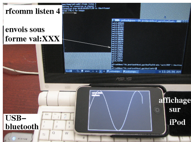
FIG. 11 – Transmission de données depuis un PC, via un convertisseur RS232-Bluetooth lui même connecté par convertisseur USB-RS232, pour affichage sur iPod. Cette application est représentative d'une application dans laquelle les données sont acquises par un microcontrôleur et transmises par liaison Bluetooth grâce au convertisseur Free2Move, les données étant émises selon un format val : valeur au travers du port série.
