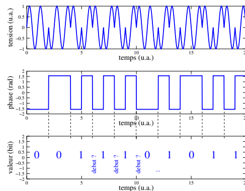
FIGURE 5: Séquence de décodage des trames : le passage du milieu au bas est conforme au Tab. 2 de [6] avec une conversion respectant le codage de Manchester différentiel.
