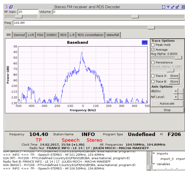
FIGURE 8 – Gauche, gr_rds en action sur France Info : la présentation est à peine plus attractive que l'exécution d'un script dans GNU/Octave et les données affichées sont sensiblement les mêmes. Nous notons à l'exécution que le nom de la station et le texte libre s'accumulent petit à petit, en accord avec la difficulté que nous observons d'obtenir une trame complète valide. Droite : la sortie de gr_rds sur Rire & Chanson, confirmant l'inclusion de l'auteur de l'émission en cours dans le titre de la station.
