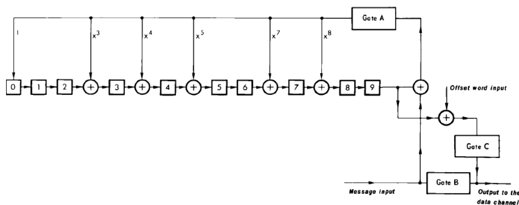
FIGURE 7 – Implémentation sous forme de registre à décalage du code correcteur d'erreur. Nous proposons l'alternative de pré-calculer les états possibles du code correcteur d'erreur pour l'implémenter sous forme d'opération matricielle, plus naturel sous GNU/Octave. Chaque symbole “ \oplus ” se comprend au sens binaire, comme un OU exclusif. Ce schéma est issu de [6, p.62].
