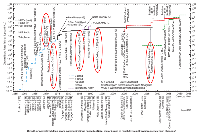
FIGURE 9: Évolution de la bande passante de communication des sondes spatiales.
