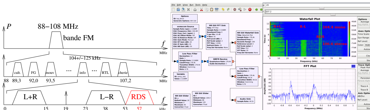
FIGURE 1 – Gauche : la bande de fréquence qui nous intéresse – RDS – se trouve à 57 kHz de la porteuse de chaque station FM : elle est donc accessible par transposition de fréquence, pour ramener le signal numérique en bande de base (autour de la fréquence nulle), après la démodulation FM de la station écoutée. Droite : les divers signaux émis par une station de la bande commerciale FM sont visibles sur le mode waterfall après le démodulateur WBPFM. Nous avons changé la fréquence en milieu d'acquisition entre une station stéréo et une station mono, qui toutes deux émettent un signal d'identification RDS.
