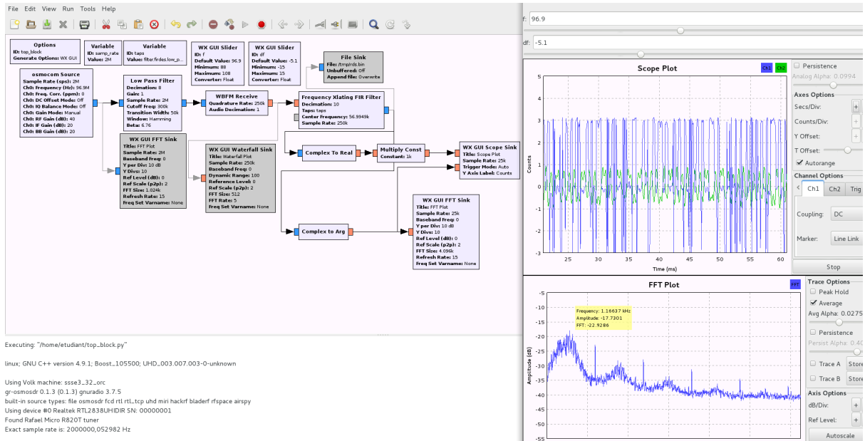
FIGURE 6 – Gauche : réception FM, suivi de l'extraction de la sous-bande RDS. En l'absence de synchronisation sur la porteuse, la phase varie trop vite pour ressembler à un signal numérique.
