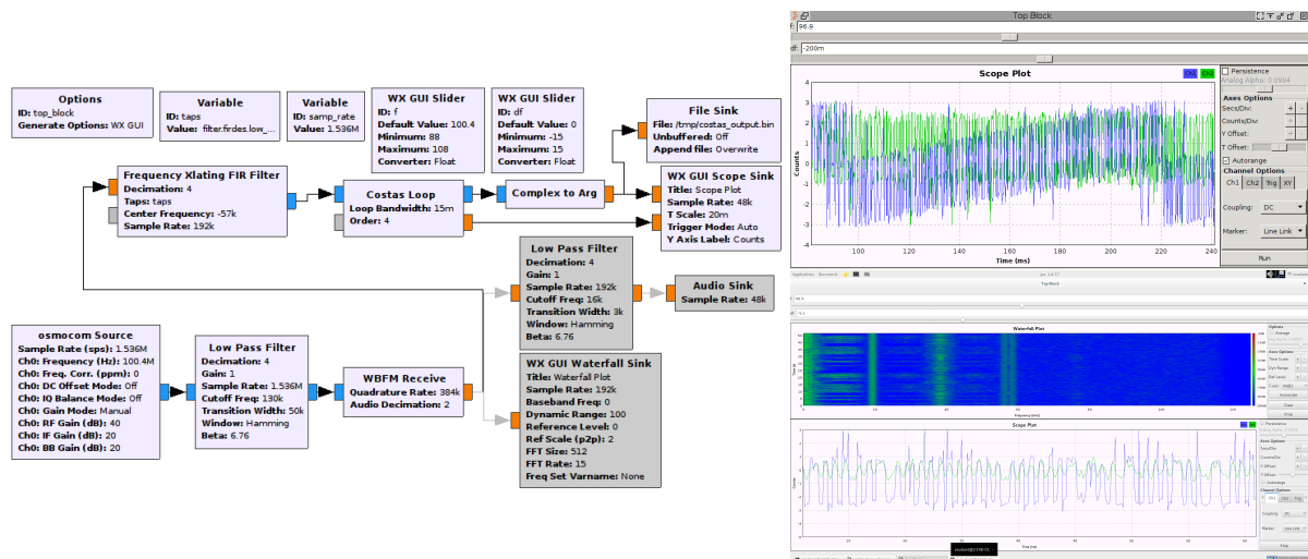
FIGURE 4 – Gauche : séquence de traitements d'un signal acquis dans la bande FM commerciale. Le mode waterfall (en bas à droite) montre clairement le pilote à 19 kHz et le RDS autour de 57 kHz. En haut à droite : en l'absence de synchronisation sur la porteuse (bleu), la phase qui encode le signal comporte encore une dérive linéaire de pente égale à l'écart entre la fréquence nominale de 57 kHz et la fréquence de l'oscillateur local numérique. L'application de la boucle de Costas (vert) élimine cet écart de fréquence : la phase représente des bits exploitables (en bas à droite en bleu).
