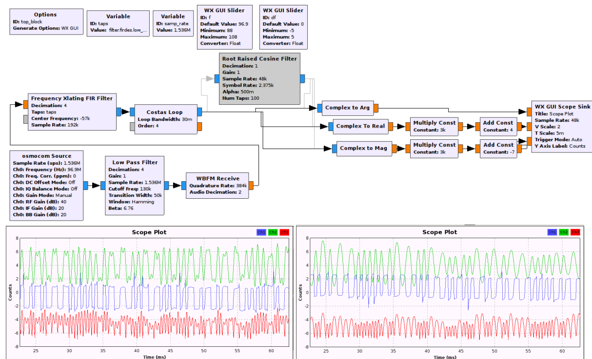
FIGURE 11 – Haut : graphique pour l'extraction des diverses composantes du signal dans la sous-porteuse RDS après asservissement de l'oscillateur par la boucle de Costas. La phase s'affichera en bleu, la partie réelle en vert, et le module en rouge. En bas : à gauche sans filtre passe bas RRC, la partie réelle présente quelques oscillations sur les symboles les plus longs. En bas à droite : un filtre RRC permet d'atténuer ces artéfacts et de rendre la partie réelle du signal exploitable. Dans tous les cas, le module (rouge) est inexploitable.
