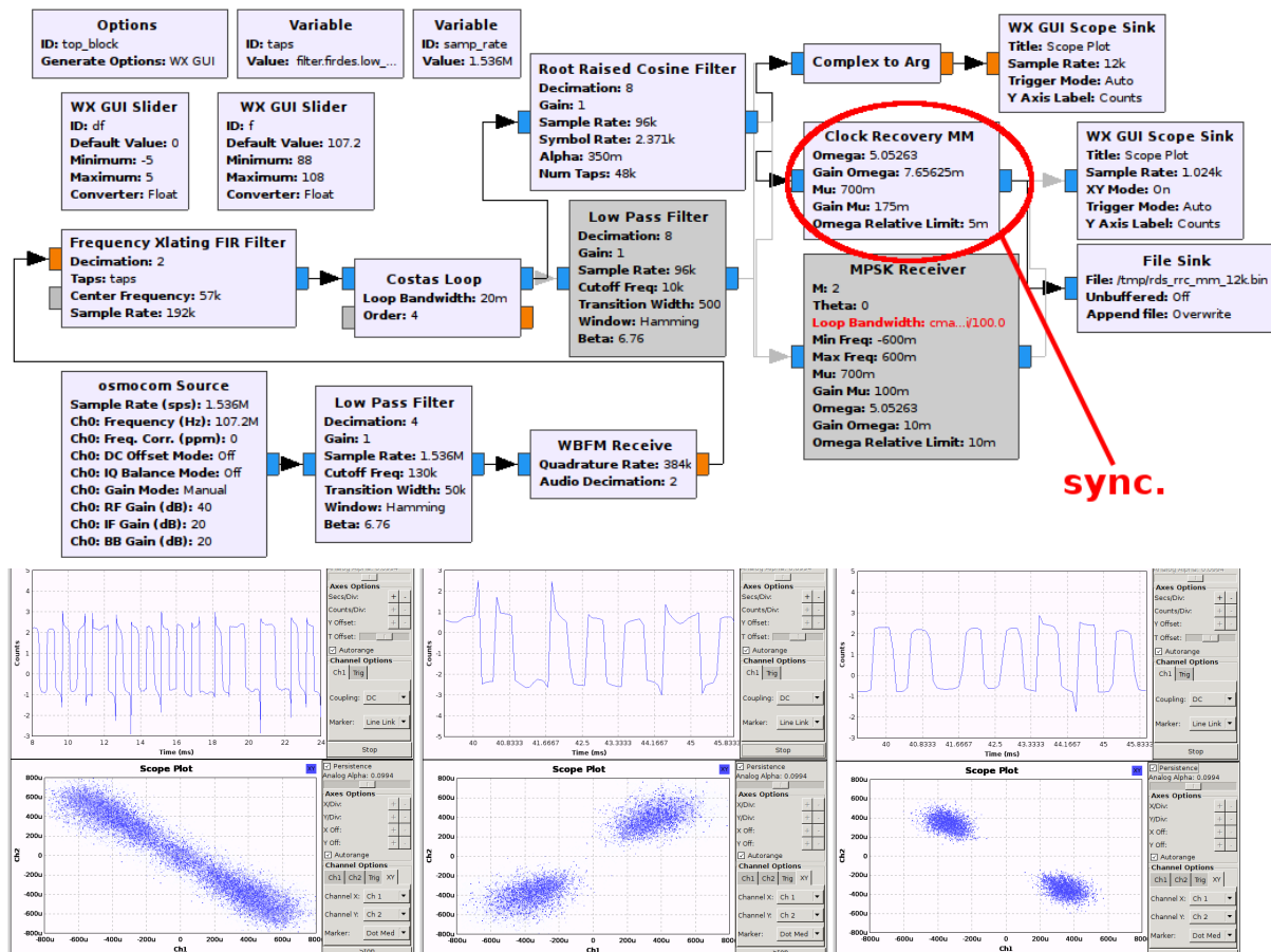
FIGURE 14 – Haut : flux de traitement, ajoutant la synchronisation du flux numérique après la synchronisation sur la porteuse (Costas). En bas : diagramme de constellation (mode XY d'un oscilloscope recevant le flux de données complexes) dans les diverses conditions – de gauche à droite, sortie de la boucle de Costas (sans synchronisation de la séquence numérique), synchronisation de l'horloge numérique après un filtre passe bas, et finalement après un filtre RRC. Deux nuages de points distincts garantissent la capacité à séparer les symboles.
