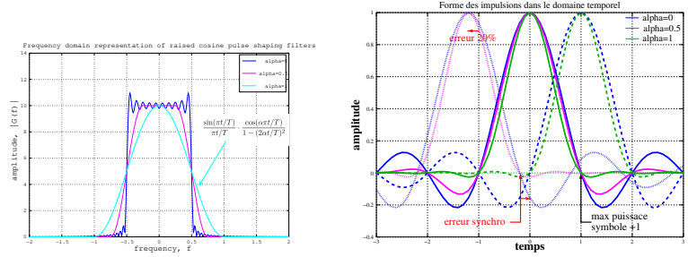
FIGURE 12: Gauche : réponse spectrale des filtres RRC avec diverses formes, du rectangle (meilleure sélectivité spectrale) au segment de fonction trigonométrique. Droite : plusieurs impulsions successives dans le temps, filtrées avec diverses formes de RRC, avec l'impulsion de gauche décalée de 20% par rapport à sa date nominale pour une transmission périodique.
