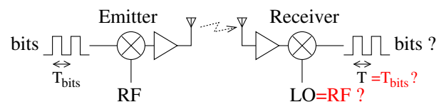
FIGURE 3: Problème de synchronisation des oscillateurs distants qui portent le signal et cadencent le débit de donnée. Le décodage ne sera fonctionnel que si les deux oscillateurs du récepteur – LO et échantillonnage de l'état de l'information numérique – sont asservis sur leurs homologues du côté de l'émetteur.
