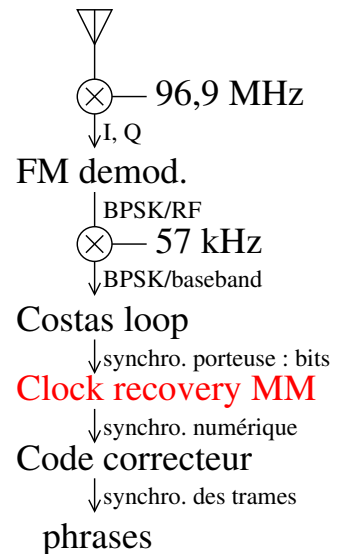
FIGURE 13: Chaîne de traitement des informations acquises depuis l'antenne pour retrouver le message (phrases) : dans cette annexe, nous nous intéressons à la synchronisation du message numérique, en rouge.
