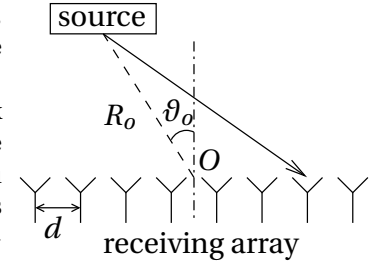
FIGURE 1: Différence de phase entre les signaux acquis par un réseau d'antennes, ici une géométrie linéaire uniformément distribuée qui facilite l'analyse de la relation entre la phase \varphi , la distance entre antennes d et la direction d'arrivée \theta_0 sous hypothèse que la distance source-réseau d'antennes R_0 est "grande" ( R_0 \gg 2(Kd)^2/\lambda pour K antennes séparées de d ) pour vérifier la condition d'onde plane incidente de longueur d'onde \lambda : \varphi = 2\pi nd\theta_0/\lambda au n ème élément.
