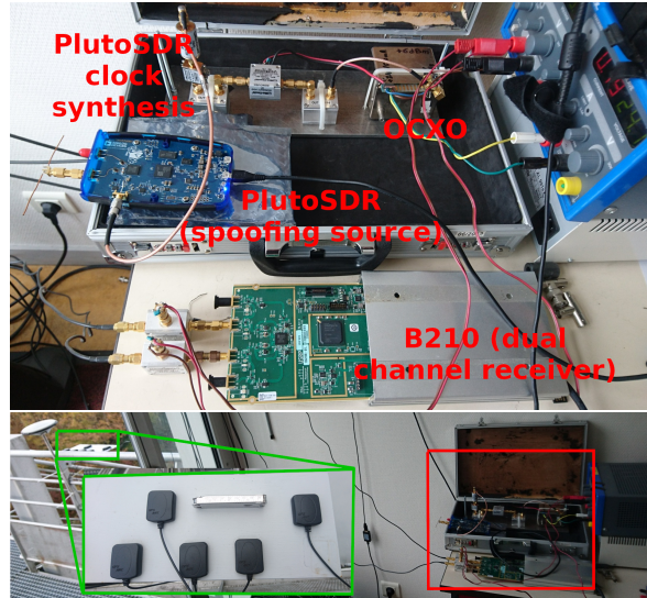
FIGURE 2 – Photo (haut) représentant le matériel utilisé pour le leurrage (PlutoSDR associé à l'oscillateur OXCXO) ainsi que le récepteur GPS (B210) connecté aux deux antennes (bas) espacées de la longueur d'onde de la porteuse à la fréquence L1 (1575,42 MHz) divisée par deux, soit 10 cm.
