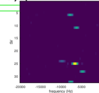
L5I-jL5Q
