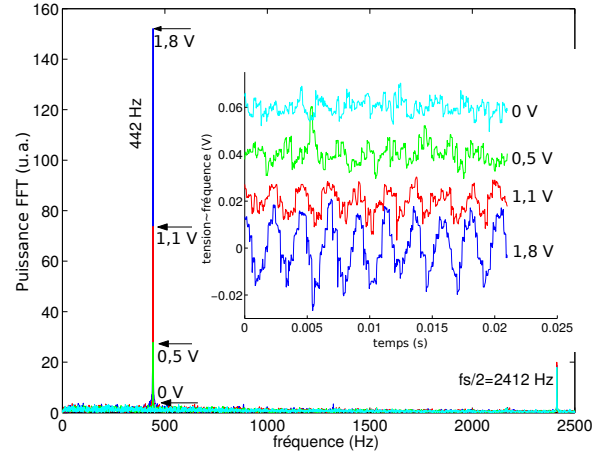
FIGURE 15. Analyse spectrale de la séquence de mesures de fréquences de résonance d'un résonateur à ondes de surface exploité comme capteur de contrainte, soudé à la base d'un diapason musical en acier inoxydable. La demi-fréquence de rafraîchissement est visible comme une raie à 2412 Hz. En insert, les mesures temporelles traitées pour fournir les spectres : les tensions indiquent l'amplitude du signal alimentant un microphone dont le solénoïde entretient la vibration du diapason.
