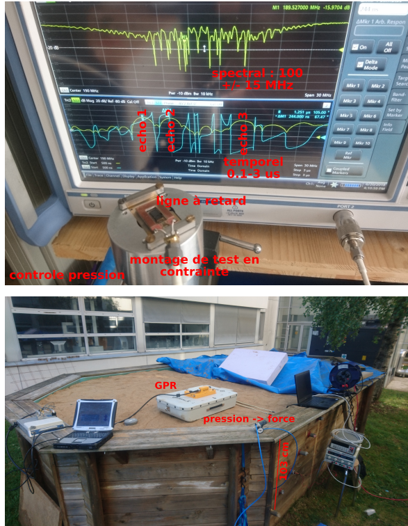
FIGURE 14. Haut : ligne à retard réflective conçue pour fonctionner dans la bande 100 \pm 15 MHz comme cible coopérative d'un RADAR de sol, montée comme capteur de contrainte sur un corps d'épreuve en acier inoxydable. Le montage de qualification visible devant l'analyseur de réseau (en haut la réponse spectrale, en bas temporelle par transformée de Fourier inverse) applique une force sur un montage 3-points en variant la pression dans un piston sans affecter le bilan de liaison radiofréquence par l'insertion de fils conducteurs entre le capteur et son environnement. Bas : environnement expérimental de qualification du capteur de contrainte pour des mesures sub-surfaces (instrumentation de tuyaux enterrés) permettant des mesures par RADAR de sol dans le sable ou le gravier de capteurs enterrés jusqu'à 1 m de profondeur.
