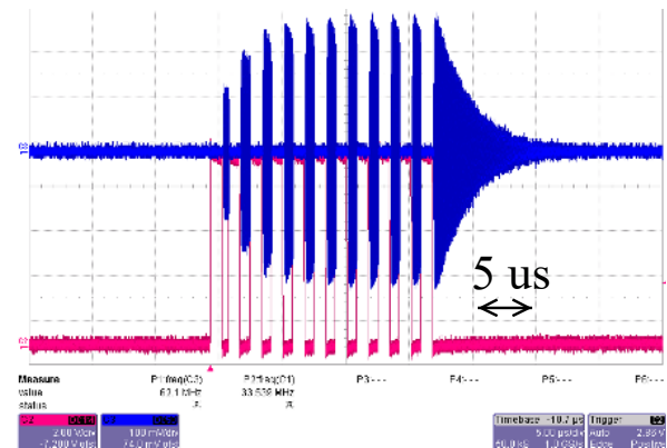
FIGURE 3. Charge et décharge d'un résonateur excité à sa fréquence de résonance. La tension aux bornes du résonateur lors de la phase de charge est coupée pour observer son évolution temporelle : dans la pratique, la porteuse est émise en continu lors de la charge pendant une durée de 5 à 10 constantes de temps du résonateur, puis coupée lors de la phase d'écoute pour observer la décroissance exponentielle du signal.
